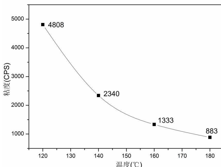
图1、EVA封箱胶粘度随温度变化图
